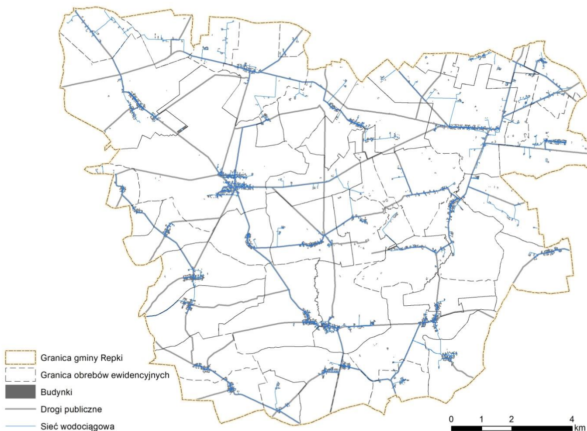
Rysunek 9. Schemat sieci wodociągowej
